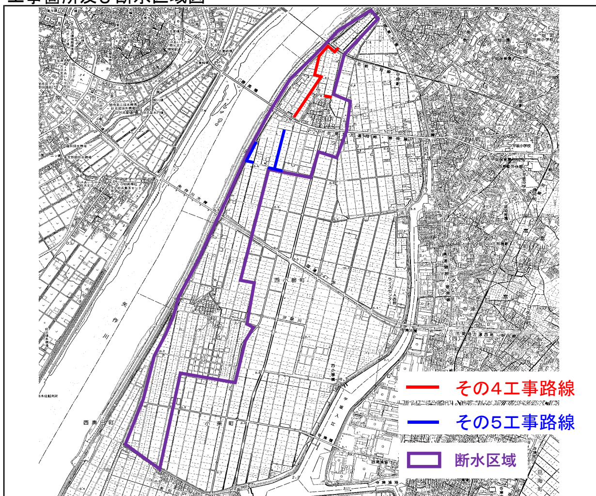
工事箇所及び断水区域図
